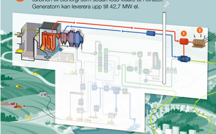
Skissen visar hur el- och värmeproduktionen går till på Sävenäs avfallskraftvärmeverk.
